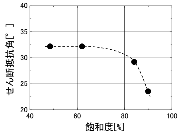
図4 せん断抵抗角と飽和度の関係
