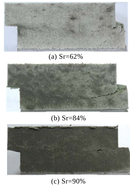
図5 各種飽和度の試験後の供試体
