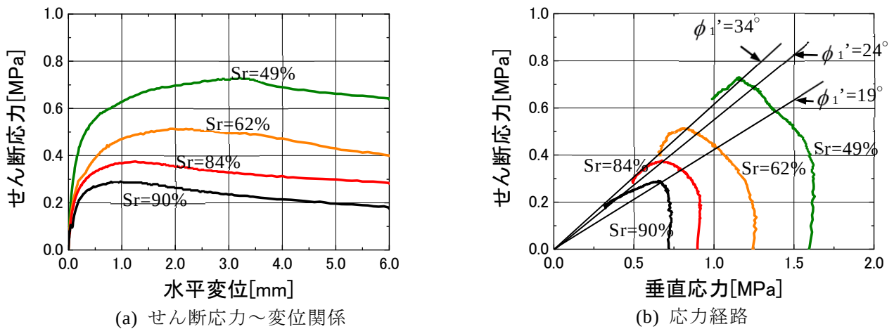
図3 各種飽和度の珪砂・ベントナイト混合体の一面せん断試験結果
