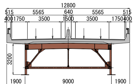
図-1 横断面図
