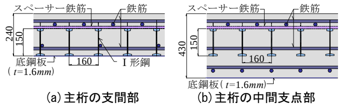
図-3 縦置き IB 床版の断面
