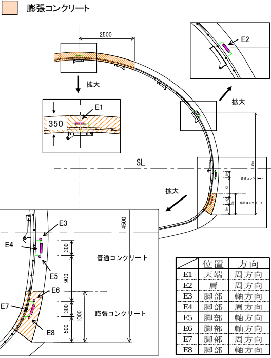
図-1 ひずみゲージ設置位置
