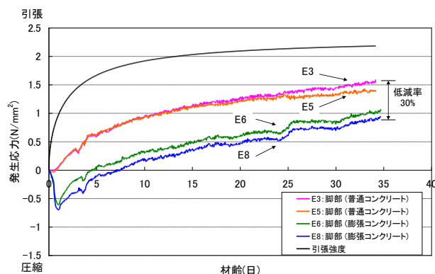
図-3 コンクリートの発生応力
