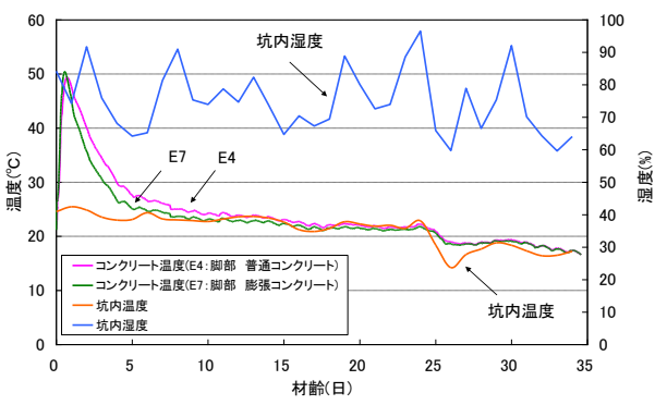
図-2 坑内環境および覆工コンクリート温度
