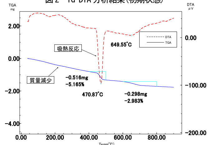
図3 TG-DTA分析結果(湧水状態1ヶ月後)
