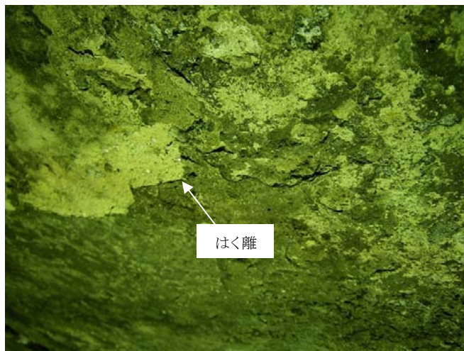
写真1 覆工内面のはく離現象
