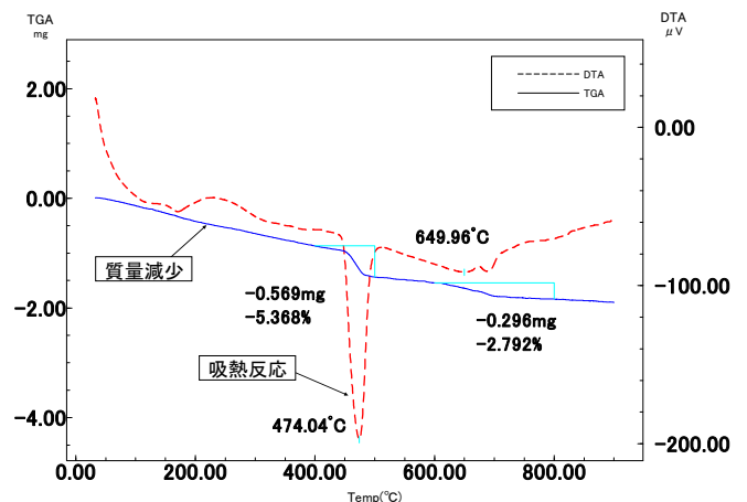
図2 TG-DTA分析結果(初期状態)
