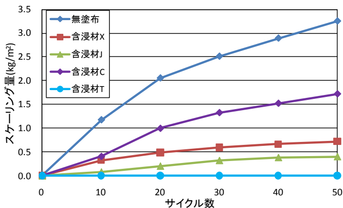
図-2 スケーリング試験結果(高炉セメント)
