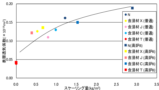
図-3 透気係数とスケールング量の関係
