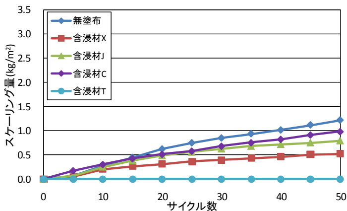
図-1 スケーリング試験結果(普通ポルトランドセメント)
