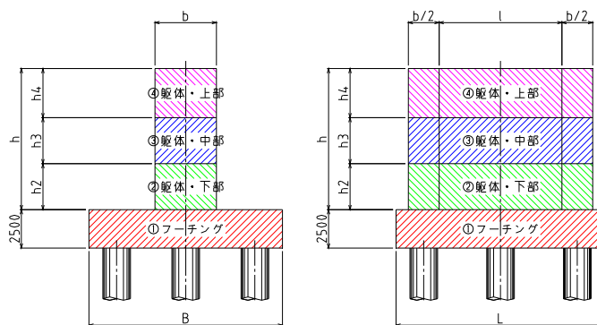
図 2 打設計画
