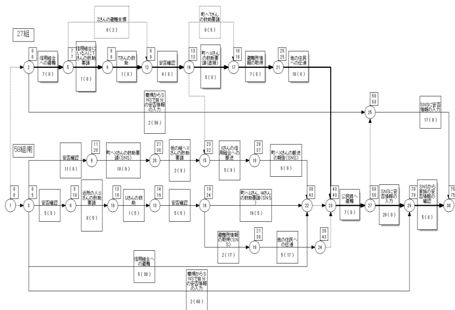
図-2 ガントチャートに基づいたアローダイアグラム
