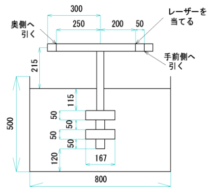
図5 実験概略図
