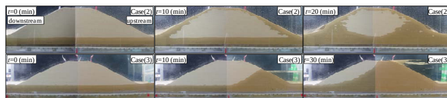
図-2 浸潤線の経時変化 (Case(2)および Case(3))
