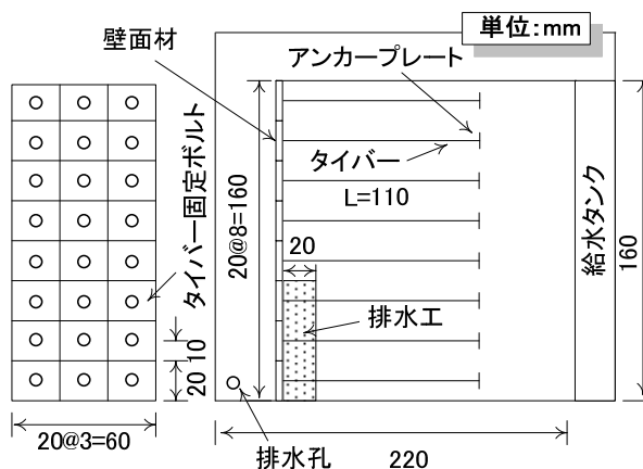
図-1 実験システム図
