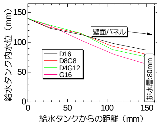
図-5 盛土内水位の比較
