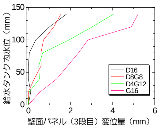
図-7 給水タンク内水位～ 壁面パネルの変位量の関係
