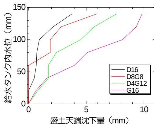
図-6 盛土天端沈下量の推移 (給水タンクからの距離：約 90mm)
