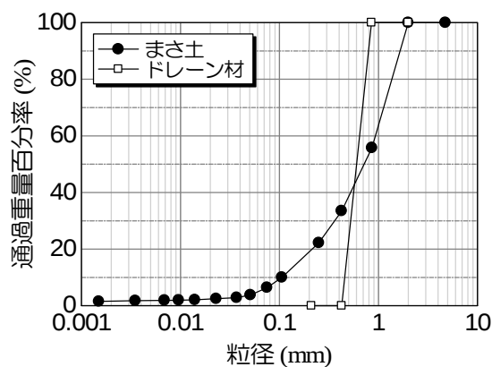
図-2 各地盤材料の粒径加積曲線
