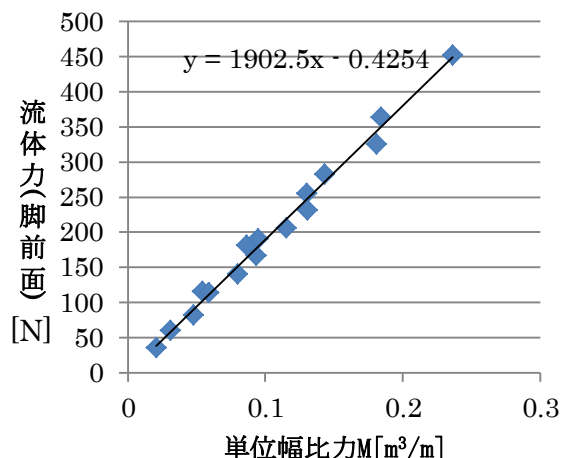
図 3. 脚前面にかかる流体力
