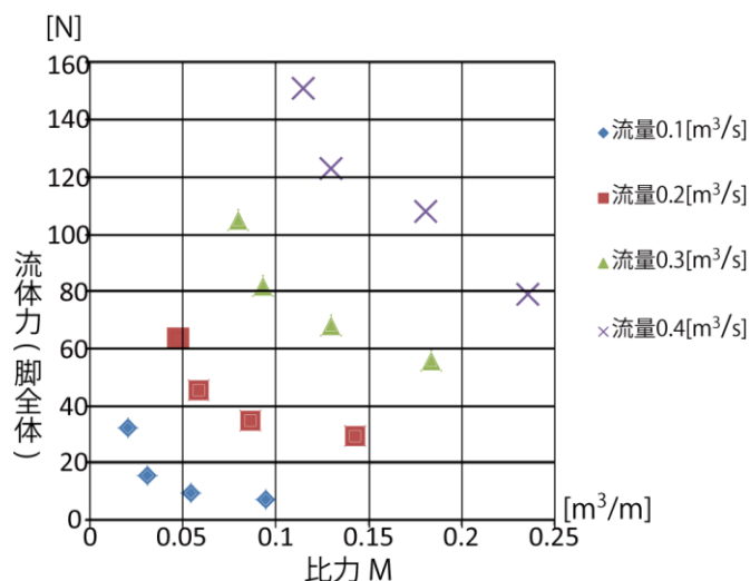
図 4. 脚全体にかかる流体力
