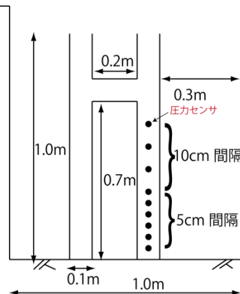
図 2. 実験模型正面図
