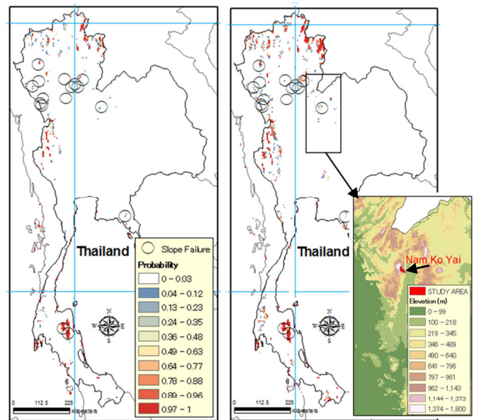
図 1 再現期間における斜面崩壊発生確率(左: 5 年, 右: 10 年), ナムコヤイ支流域の位置と標高分布(右図の拡大図)
