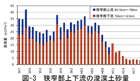
図-3 狭窄部上下流の浚渫土砂量
