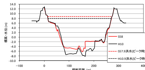
図-7 76.5km 地点の横断面図と痕跡水位
