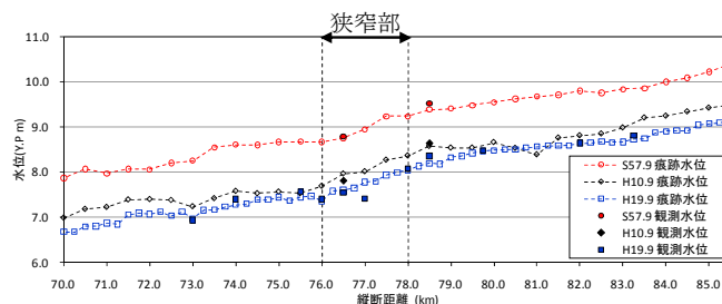
図-4 各洪水の痕跡水位縦断図と観測水位
