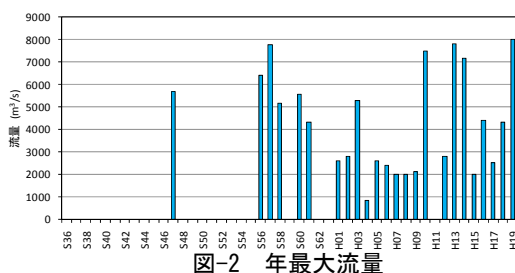
図-2 年最大流量
