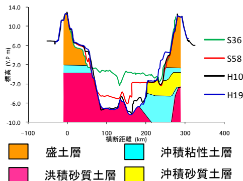
図-9 76.5km 地点の地質横断面図
