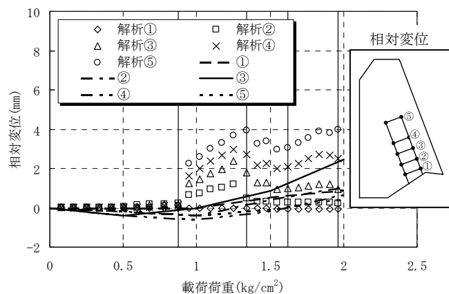
図7 基礎岩盤の相対変位の比較
