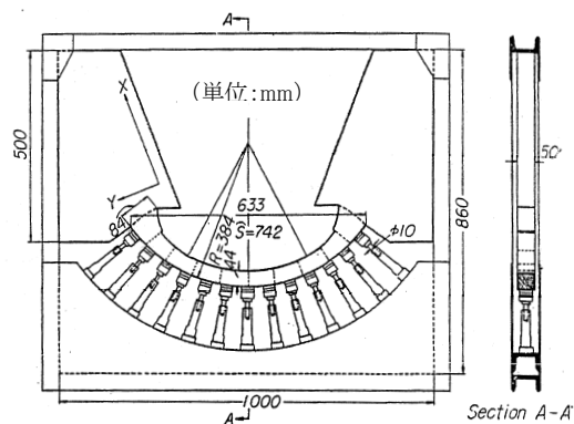
図1 試験体と加力フレームの概要
