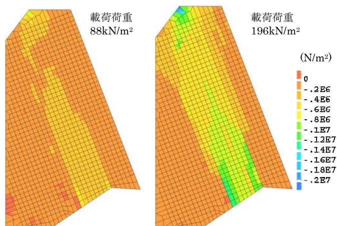
図6 最小主応力分布
