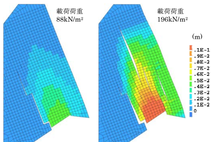
図5 変形分布
