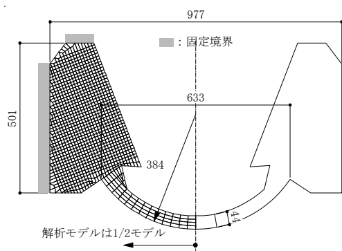
図4 解析モデル
