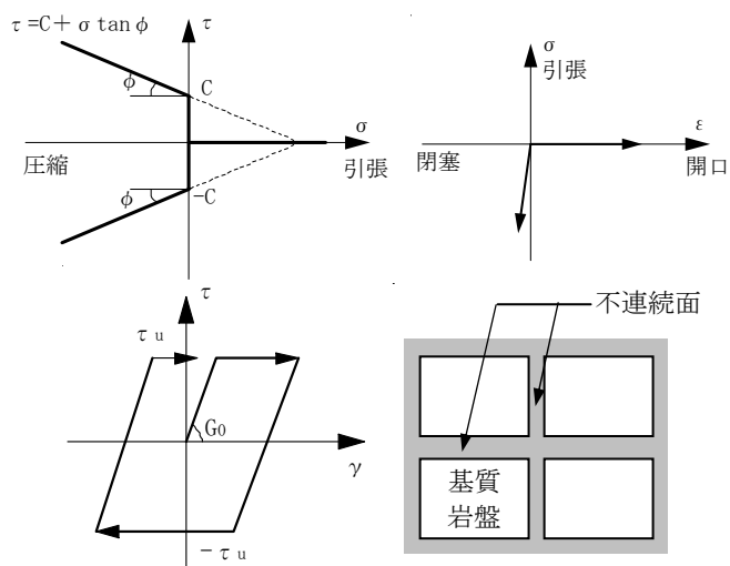
図3 不連続面の構成モデル
