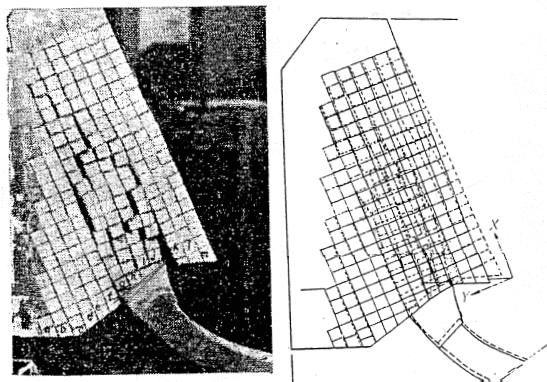
図2 試験体の破壊状況
