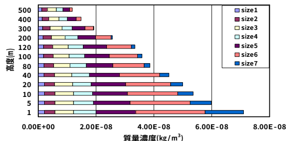
図-1 海面直上での質量濃度分布 2),3)
