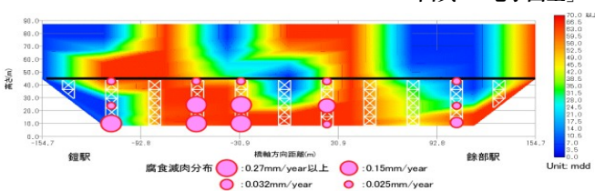
図-3 7 風向についての日平均飛来塩分量分布
