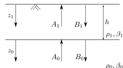
図2 2層地盤モデル
