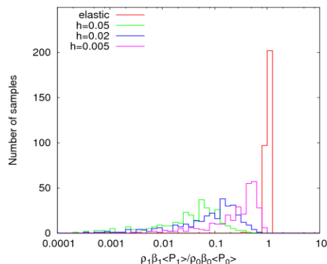
図4 減衰定数 h による導入
