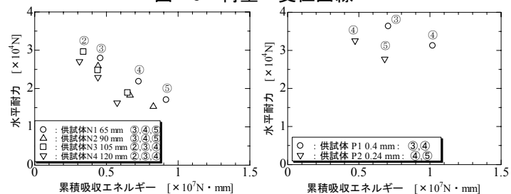
(a) 横拘束筋拘束 供試体 N
