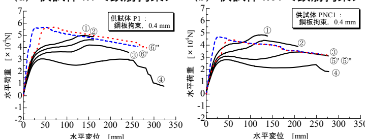
(c) 供試体 P1 <鋼板拘束>
