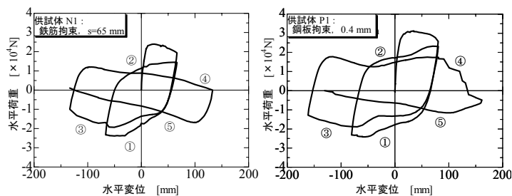
(a) 供試体 N1 <鉄筋拘束> (b) 供試体 P1 <鋼板拘束>
