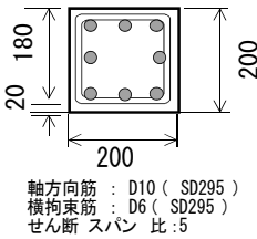
図-1 供試体断面図
