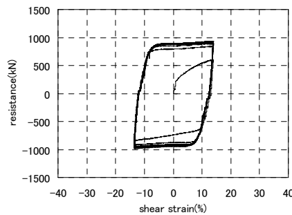
図7 一定変位試験 12.8% (L100-24)
