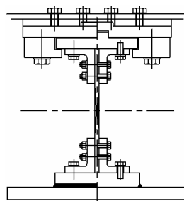
図1 LSDの構造(LY100-24-12試験体)
