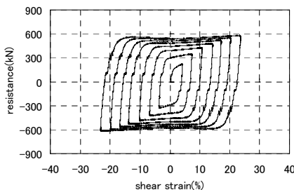
図3 変位漸増試験(L100-18)
