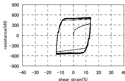
図4 一定変位試験12.8%(L100-18)
