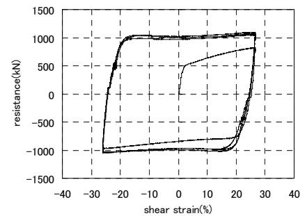
図8 一定変位試験 25.6% (L100-24)
