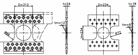
図1 LSDの構造(LY100-24-12試験体)
