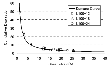
図11 損傷度評価
