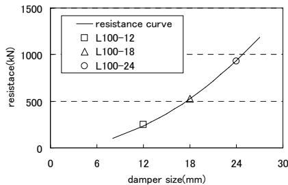
図9 LSD の形状と抵抗力 (12.8%)
