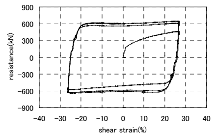
図5 一定変位試験25.6%(L100-18)
