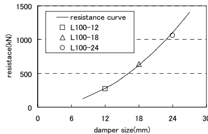
図10 LSD の形状と抵抗力 (25.6%)
