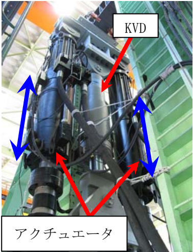
写真-1 試験装置概要
