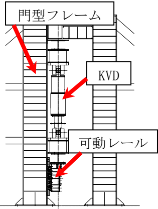
図-2 外観図
