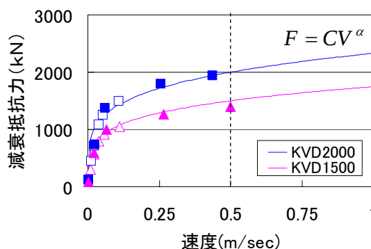
図-6 設計曲線との比較
