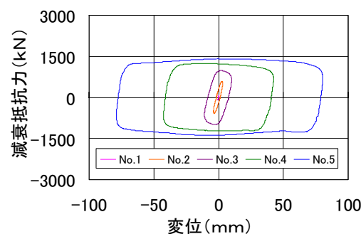
図-5 KVD1500 履歴図
