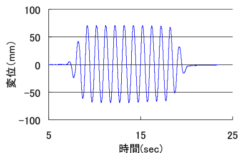
図-3 時刻歴応答(変位)一例
