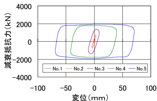
図-4 KVD2000 履歴図
