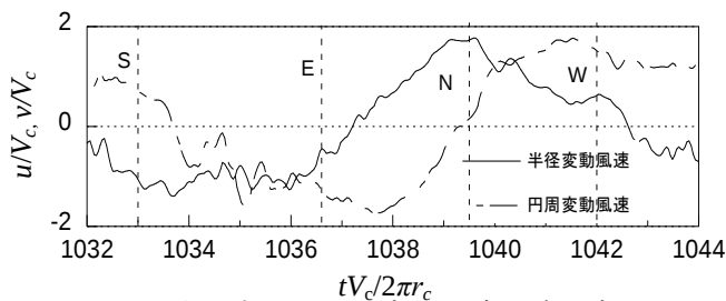
図5 中心点における変動風速の時間変化
