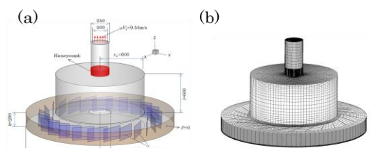
図1 数値解析モデルの(a)鳥瞰図と(b)格子分布
