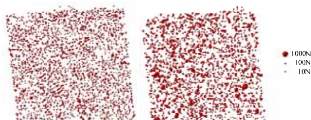
図-5 接触力図
