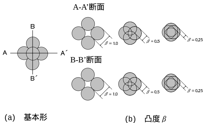
図-3 集合体要素モデル
