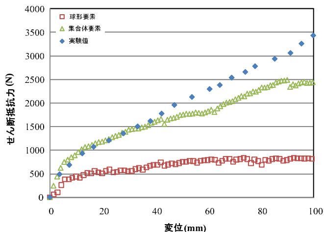
図-4 せん断抵抗力～変位関係
