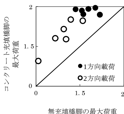
図4 最大荷重( H_m/H_0 )
