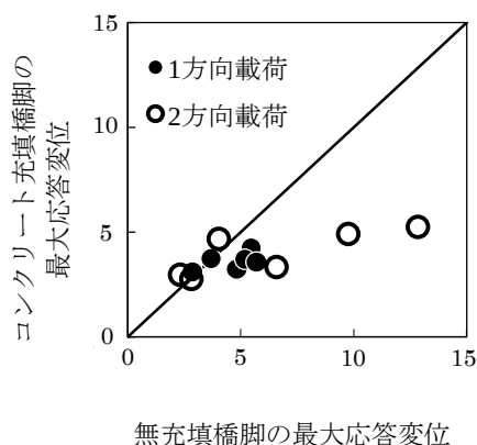
図2 最大応答変位( \delta_{max}/\delta_0 )
