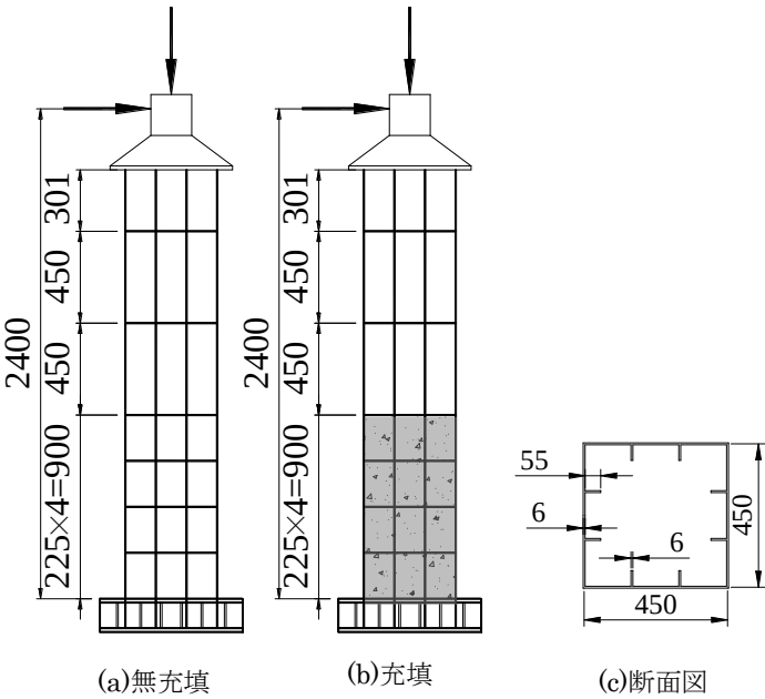
図 1 実験供試体寸法
