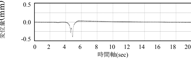
(1)床版相対変位波形(大型車通過時)
