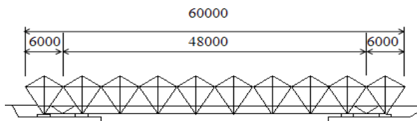
図-1 側面図
