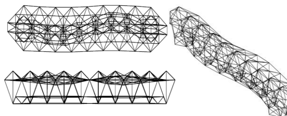
図-7 振動モード例
