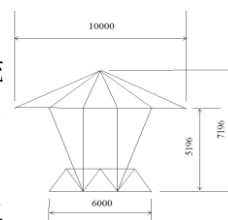
図-2 断面図
