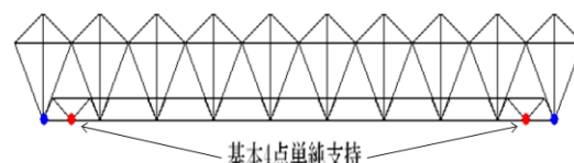
図-6 支点拘束条件側面図
