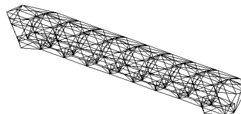
図-5 3次元構造解析モデル
