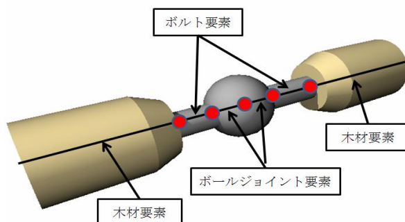
図-4 ボールジョイント部のモデル化
