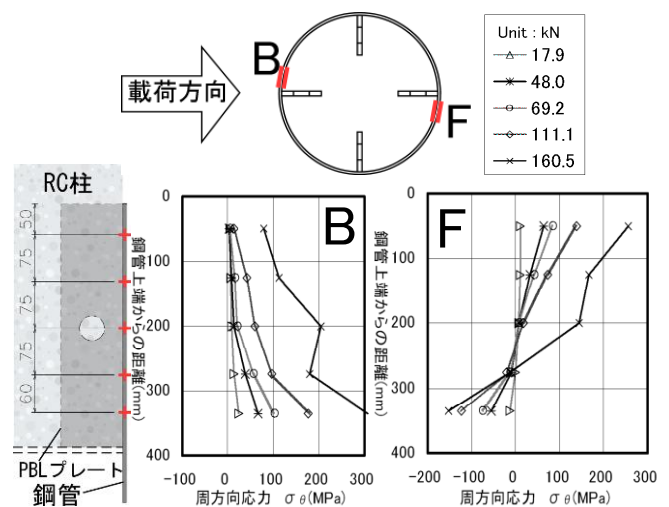
Fig.3 周方向応力分布
