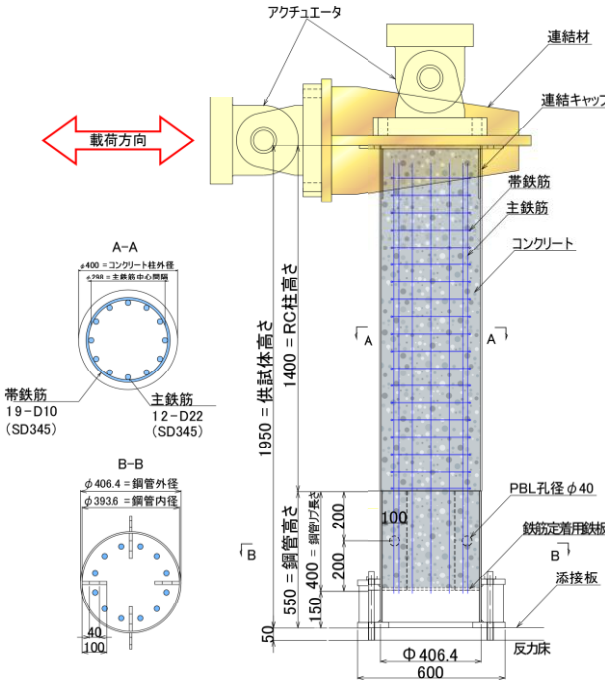
Fig.1 供試体形状
