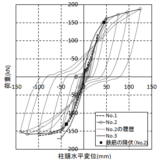
Fig.2 荷重-柱頭水平変位包絡線
