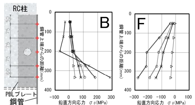
Fig.4 鉛直方向応力分布
