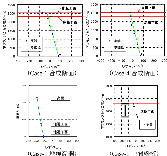
図-5 軸方向ひずみ分布
