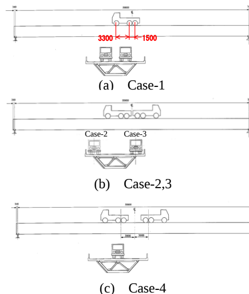
図-3 載荷パターン
