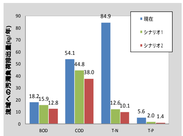
図-4 水域への汚濁負荷排出量試算結果
