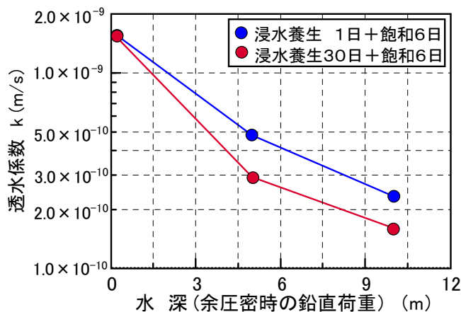
図-2 充填材の透水係数
