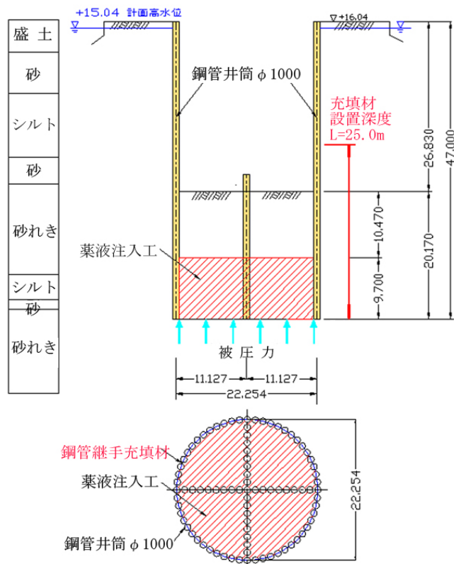
図-3 鋼管矢板基礎工 断面図
