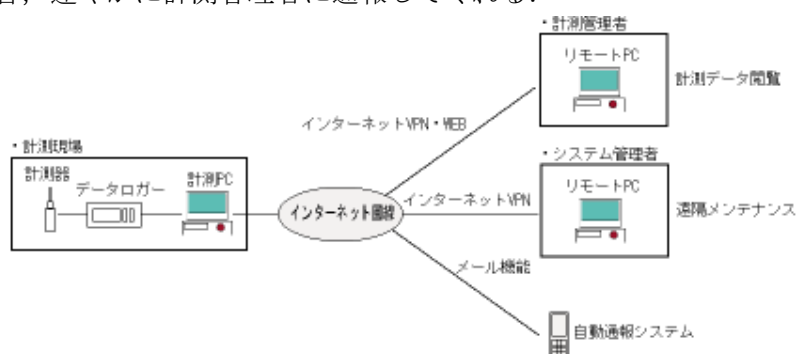
図 3-1 インターネットを利用した計測システム図
