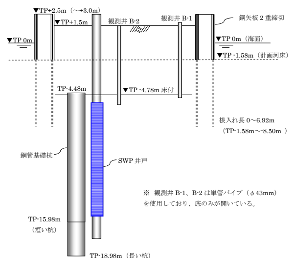
図2 SWP 井戸等の断面模式図
