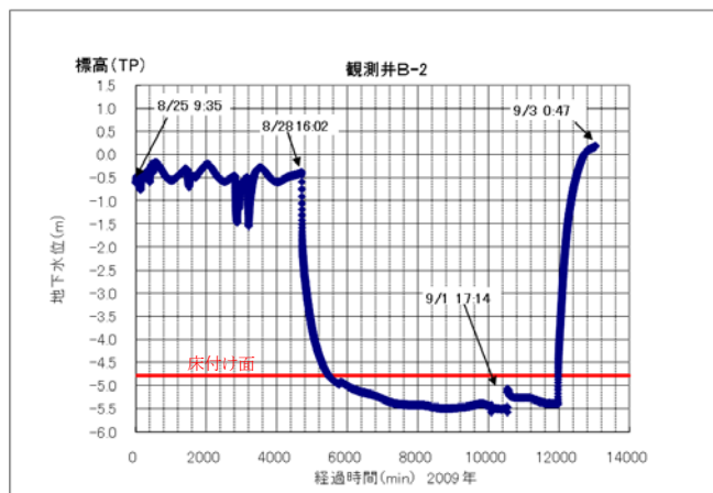
図4 観測井 B-2 の地下水位変化図
