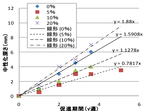
図3 促進中性化試験結果
