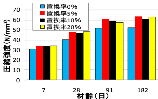
図1 圧縮強度試験結果
