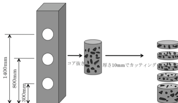
図-2 実験供試体概要
