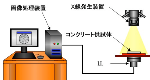
図-1 X線造影撮影の概要
