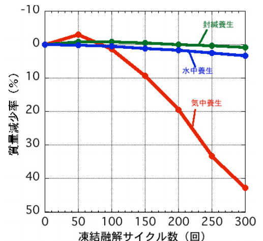
図-4 凍結融解サイクル数と質量減少率との関係
