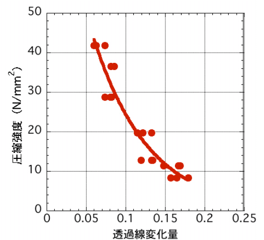
図-2 圧縮強度と透過線変化量との関係 (高炉)
