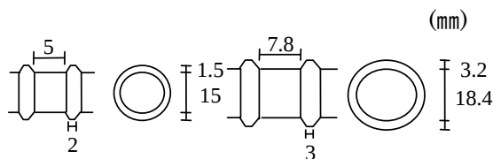
図-2 模擬異形鉄筋の形状
