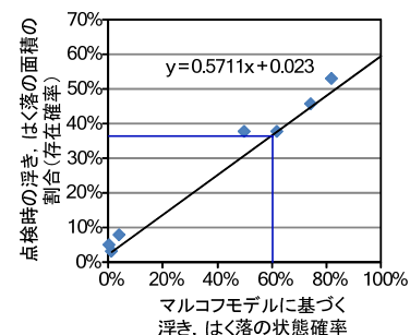
図-4.2 浮き、はく落の状態確率と存在確率の関係
