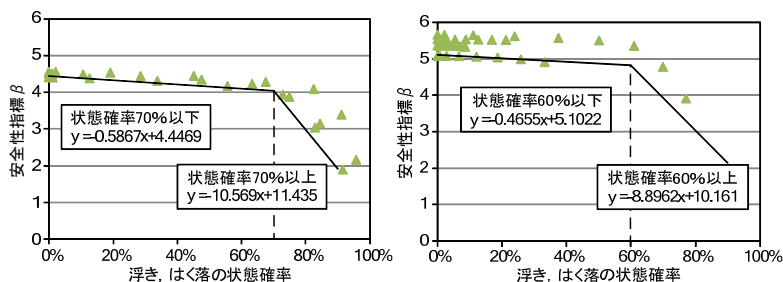
図-4.1 安全性指標 \beta と浮き、はく落の状態確率の関係式
