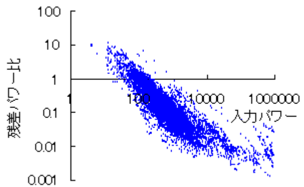
図4 入力信号のパワーと残差パワーの比率
