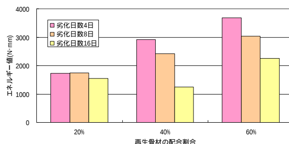
図-5 配合割合とエネルギー値の関係
