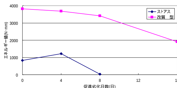
図-4 劣化日数とエネルギー値の関係
