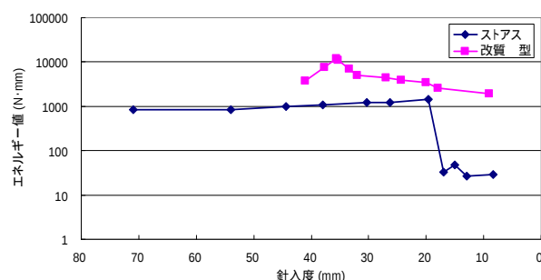
図-3 針入度とエネルギー値の関係
