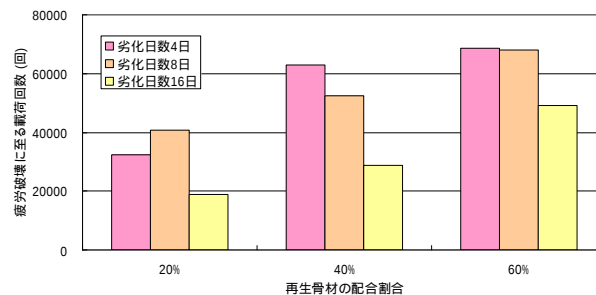
図-2 再生混合物の破壊に至る載荷回数の比較
