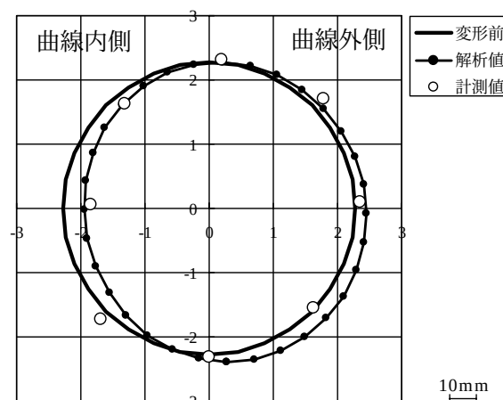
図-4 セグメント断面変位 (坑口側より切羽側を見た状態, 変位 40 倍)
