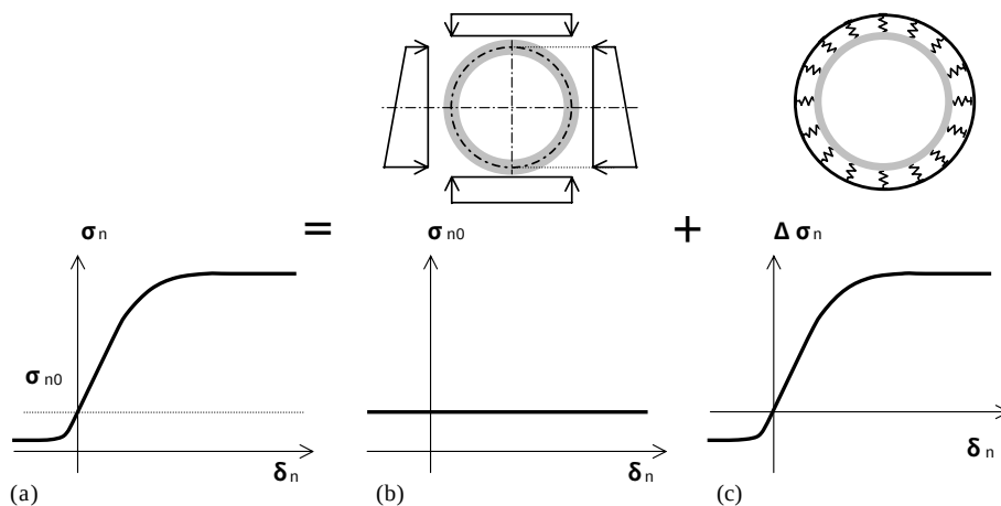
図-3 地盤とセグメントの相互作用の評価
