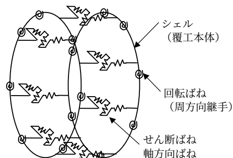
図-2 はりばねモデル
