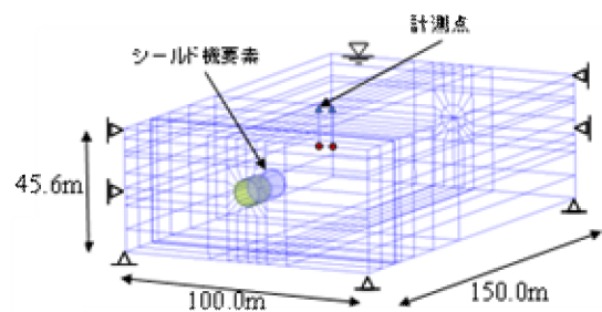
図-2 千駄ヶ谷工区メッシュ
