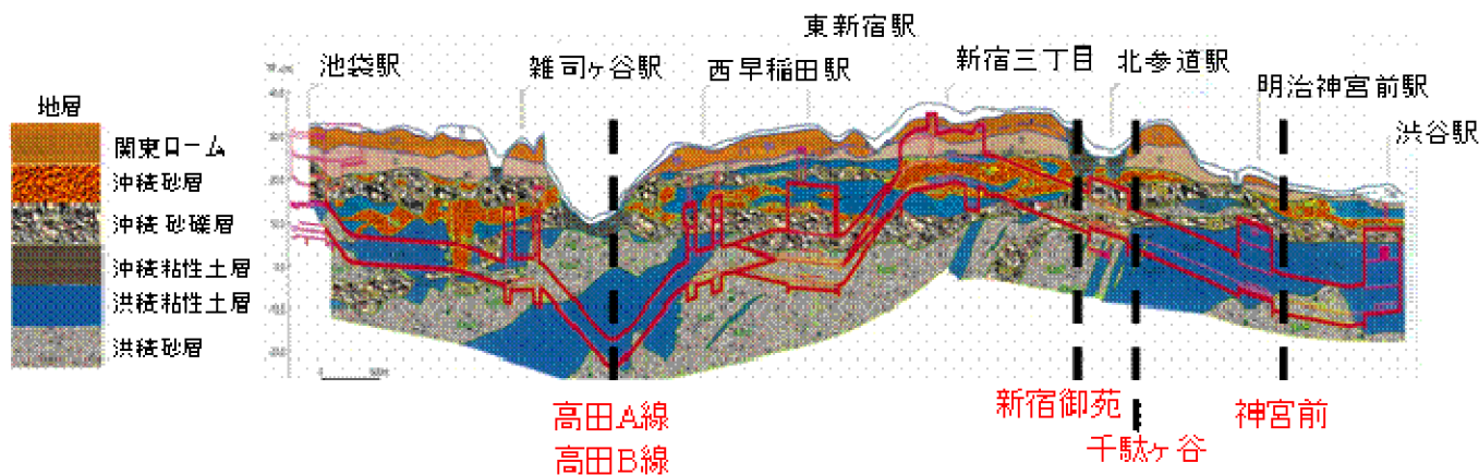
図-1 副都心線土質横断面
