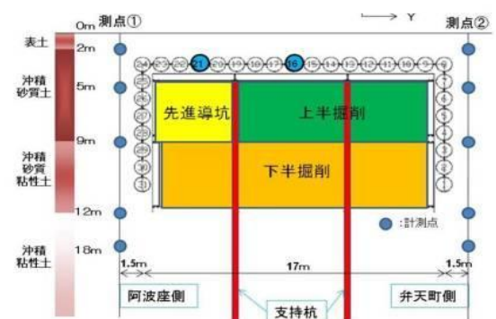
図 2.2 掘削断面図
