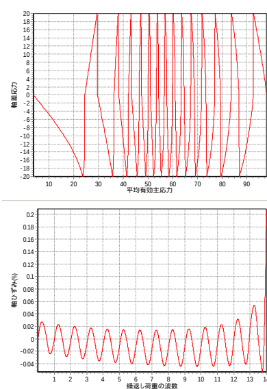
図-4 要素試験シミュレーション結果(せん断応力比 0.10)
