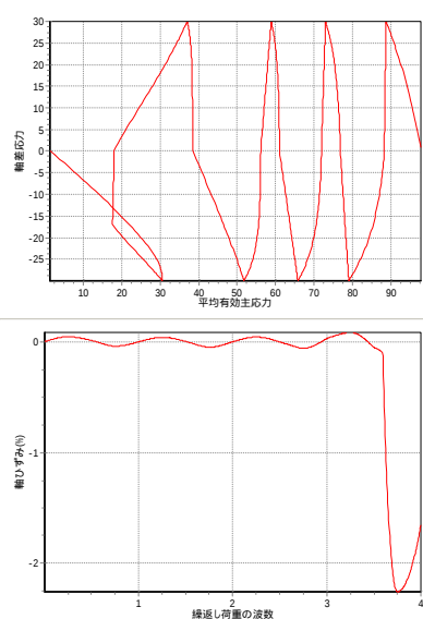
図-3 要素試験シミュレーション結果(せん断応力比 0.15)
