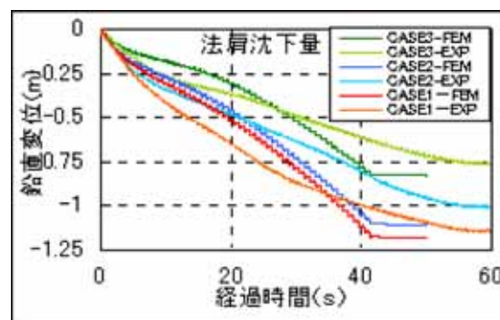
図-5 法肩沈下量の比較
