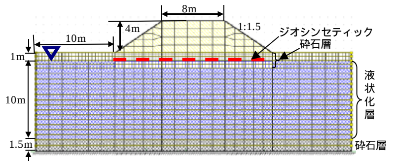
図-2 要素分割図(CASE3)
