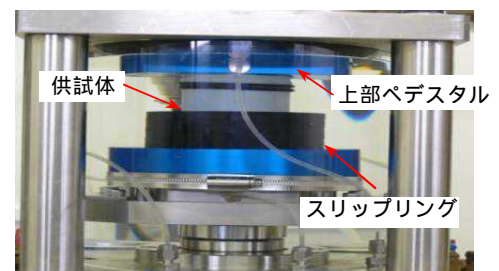
写真 1 単純せん断試験機のセル内
