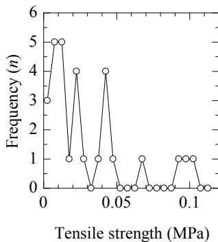
図 4 背面部の引張応力
