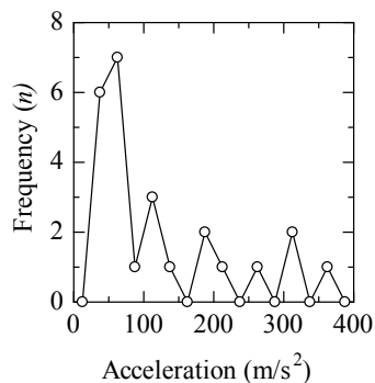
図 7 耐加速度の頻度分布
