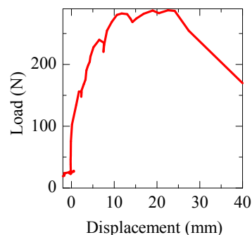
図 3 荷重-変位線図の例
