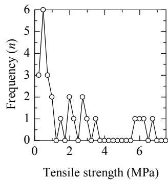
図 5 曲げ引張応力の頻度分布
