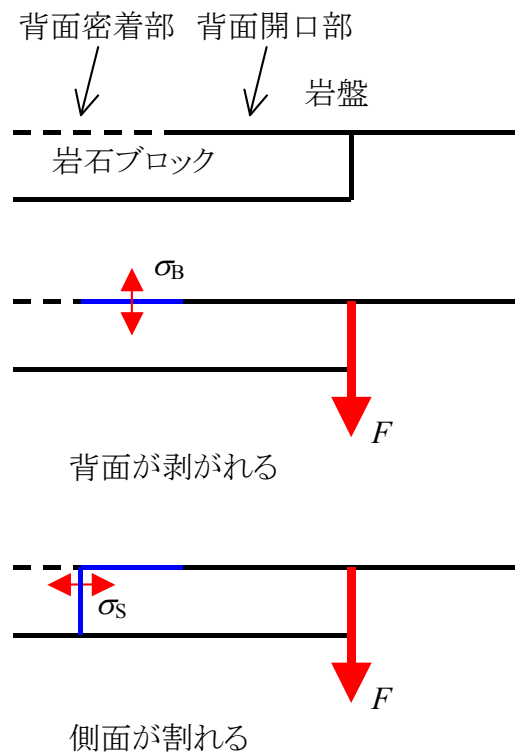
図 6 岩盤の破壊過程
