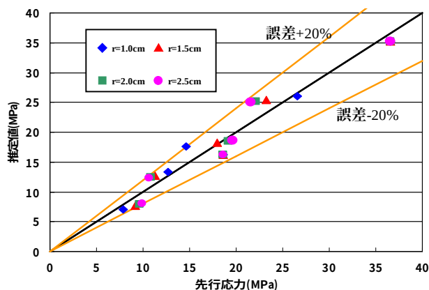
図-5 先行応力と推定値の関係
