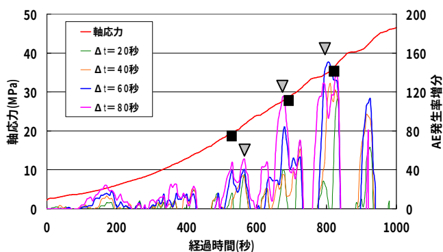
図-4 AE 発生率増分(パターン B)
