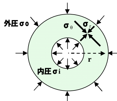
図-1 供試体断面図
