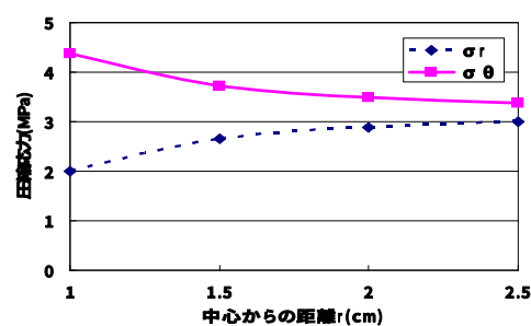
図-2 中空円筒供試体の応力分布
