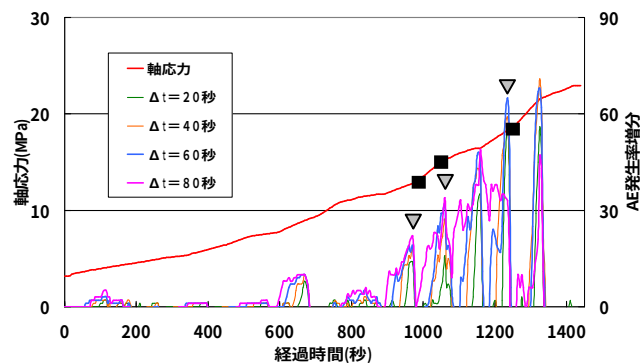
図-3 AE 発生率増分(パターン A)
