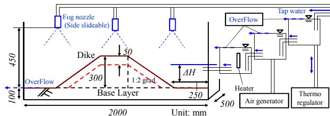
図-1 実験装置
