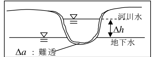
図-2 河川メッシュ上の鉛直浸透量算定
