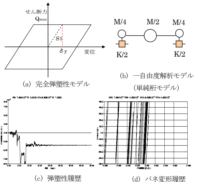
図2 1自由度解析モデル及び応答履歴
