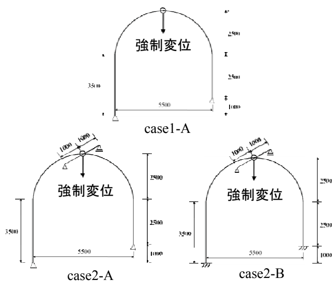
図6 パイプハウスの解析モデル
