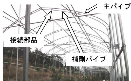
図3 主パイプに接続された補剛パイプ
