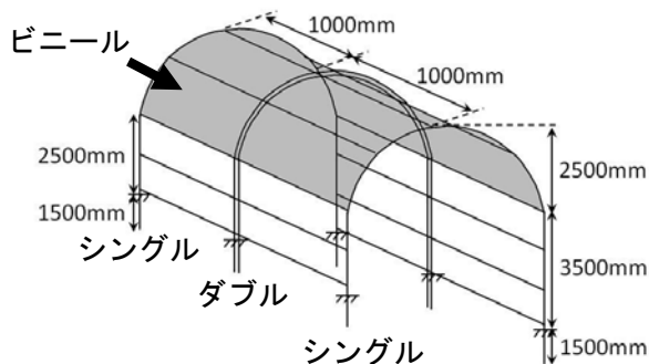
図1 実験に使用した園芸用ハウス
