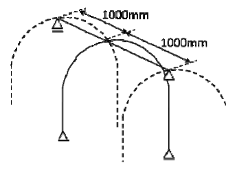
図5 奥行きを考慮した場合のモデル
