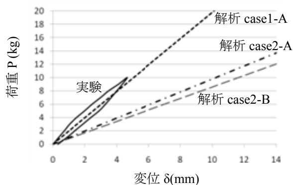
図7 シングルの荷重-変位関係
