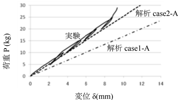
図8 ダブルの荷重-変位関係
