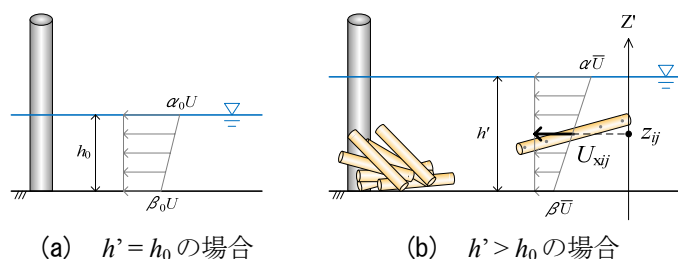
図-1 流速分布モデルの概要
