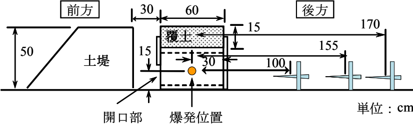
図-2 実験の概要
