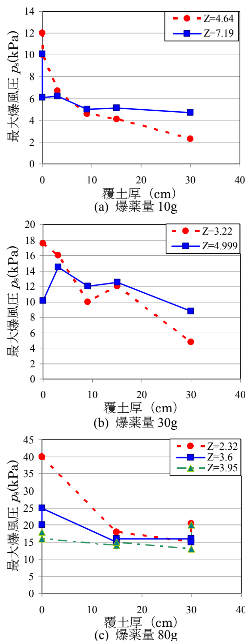
図-3 爆風圧～覆土厚関係
