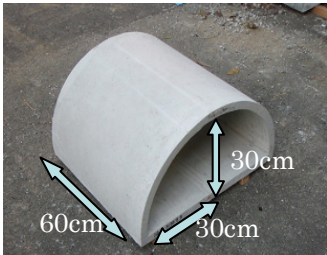
図-1 コンクリートアーチ試験体
