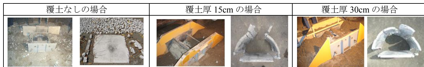
写真-1 覆土厚による破壊状況の相違 (爆薬量 80g)
